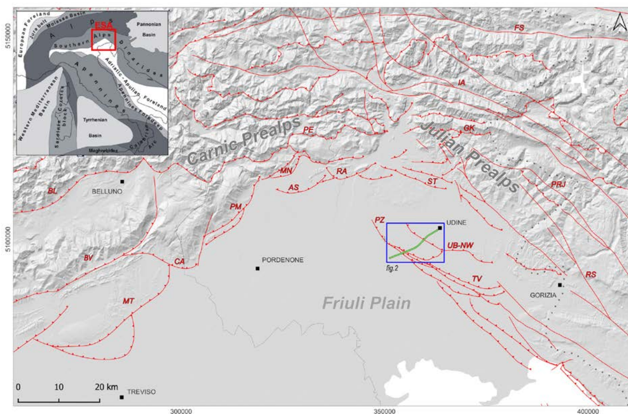
Figure 1 Structural sketch map of Eastern Southern Alps. The green line represents the measured high-precision IGM levelling line number 110; blue box represents the area mapped in Figure 2. Faults acronyms: AS: Arba-Sequals th., BL: Belluno th., BV: Bassano-Valdobbiadene th., CA: Cansiglio th., FS: Fella-Sava fs., GK: Gemona-Kobarid th., IA: Idrija-Ampezzo fs., MN: Maniago th., MT: Montello th., PE: Periadriatic th., PM: Polcenigo-Montereale th., PRJ: Predjama f., PZ: Pozzuolo ts., RA: Ragogna th., RS: Rasa f., ST: Susans-Tricesimo th., TV: Trivignano th., UB-NW: Udine-Buttrio NW th. RS: EPSG 6708.
